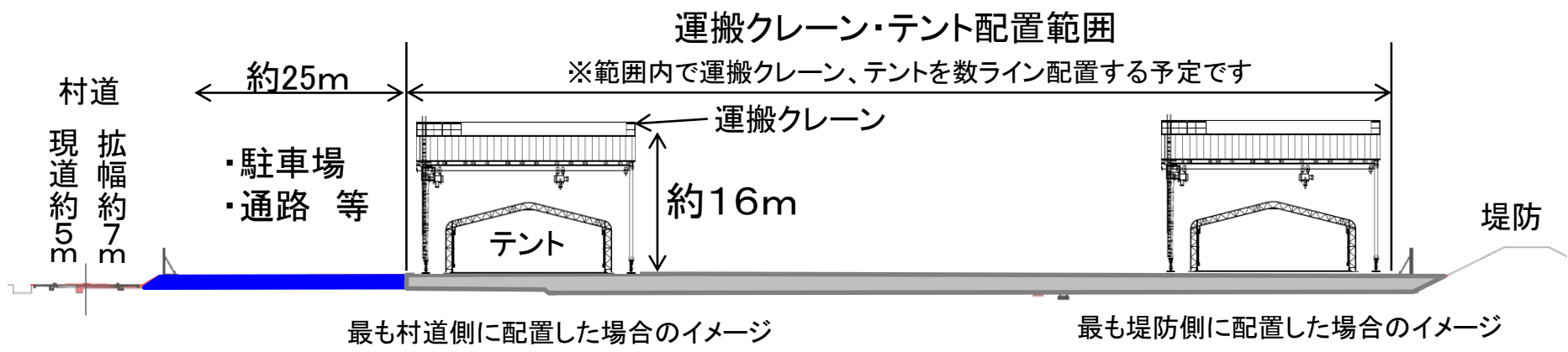
A-A' 断面図(縦横比1:1)
