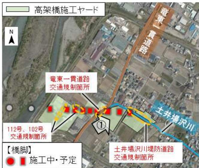
工事箇所全体図
