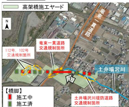
工事箇所全体図
