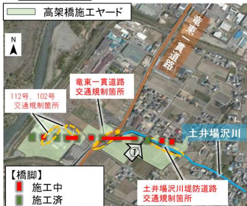
工事箇所全体図
