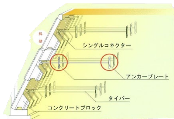
斜壁多数アンカー
