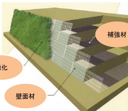
ジオテキスタイル補強土壁
