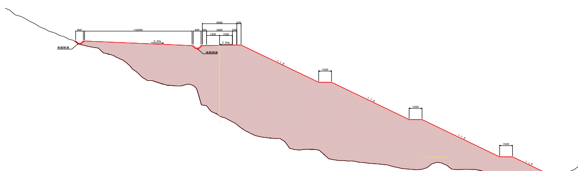
標準断面図
