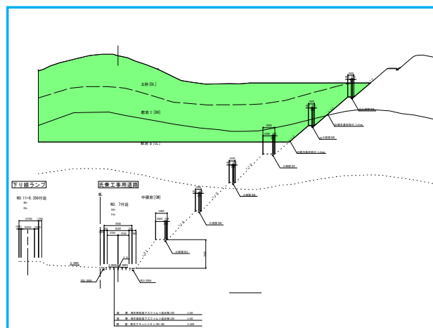
道路土工_標準図
