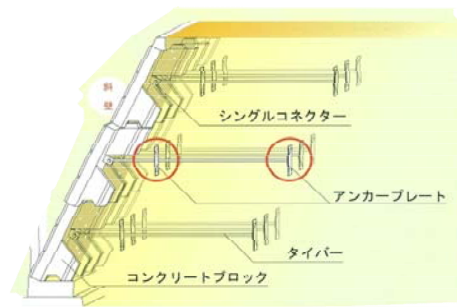
【斜壁多数アンカー】
