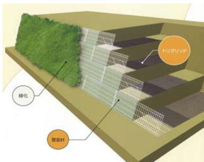
【ジオテキスタイル補強土壁】
