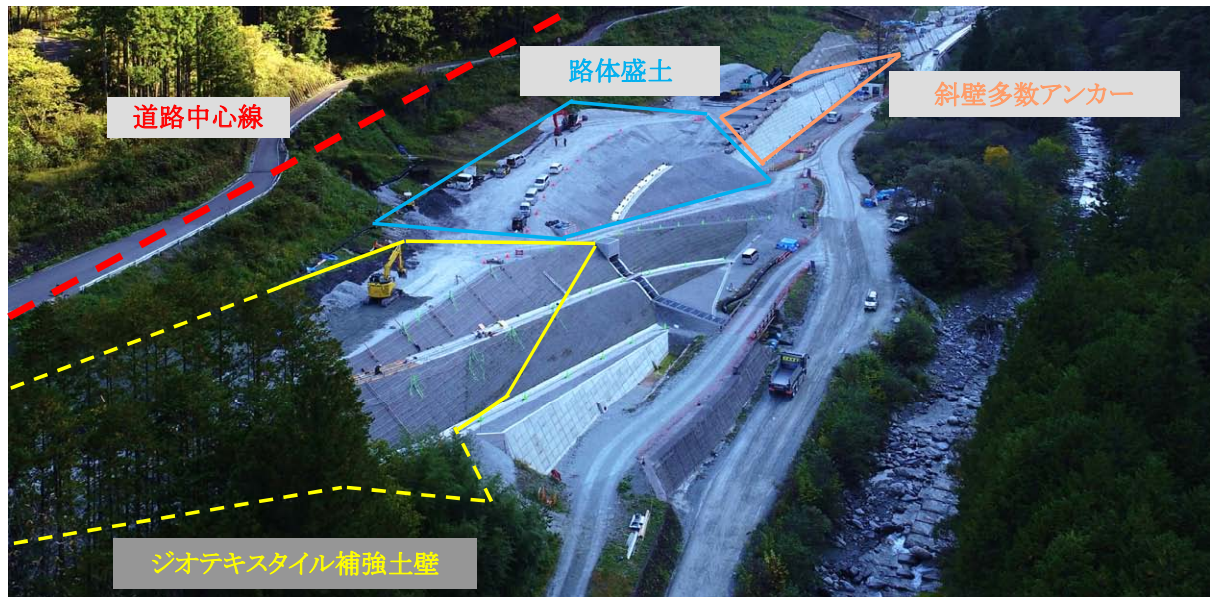
【ジオテキスタイル補強土壁】
