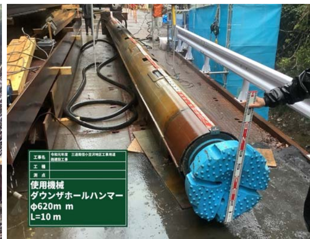
【削孔用大型ビット】
