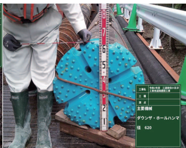
【削孔用大型ビット】
