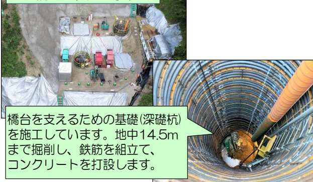
A1橋台 深礎工事状況
