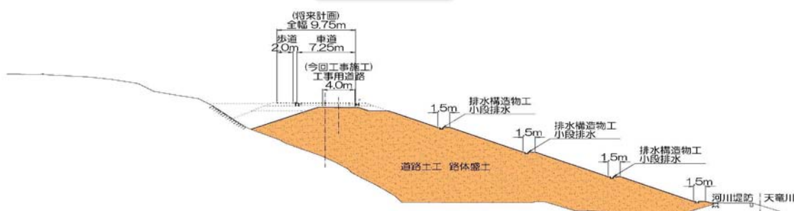
横断面図
