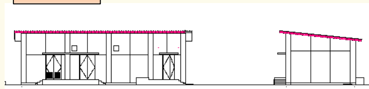
主電気室 立面図
