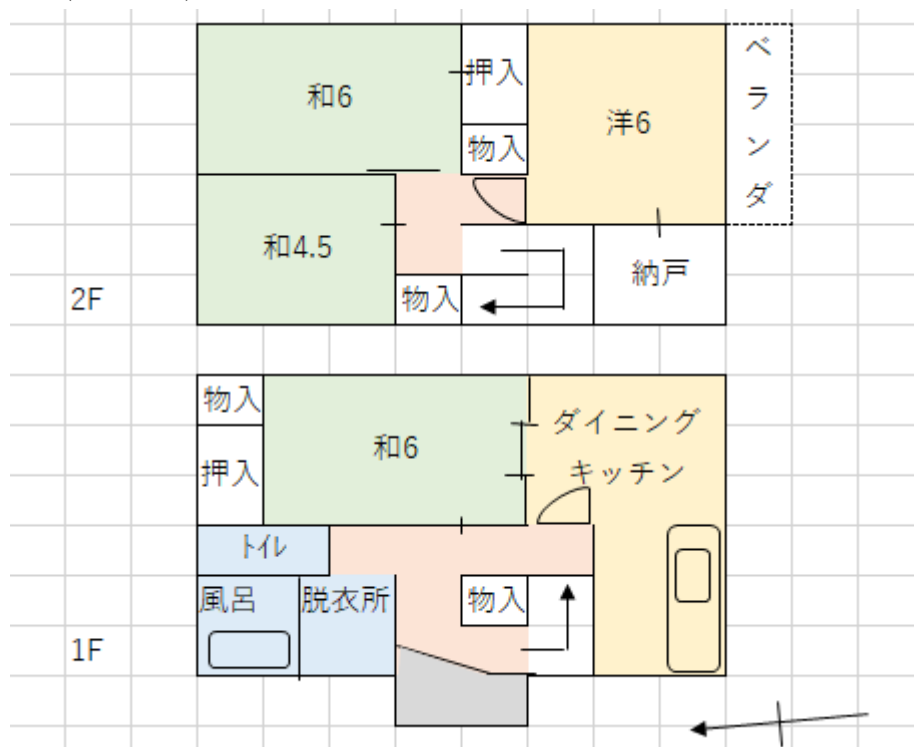
間取り図 (イメージ)
